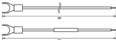
Maßzeichnung Kabel DFA 2 - RC 100
