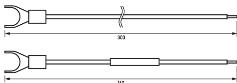
Maßzeichnung Gruppenansicht
