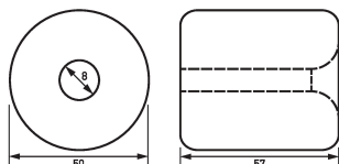
Maßzeichnung Gruppenansicht
