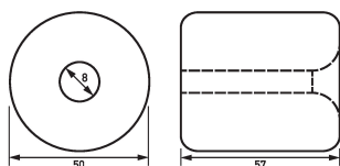
Maßzeichnung Gegengewichte GGW
