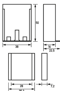
Maßzeichnung Gruppenansicht
