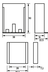
Maßzeichnung Gruppenansicht
