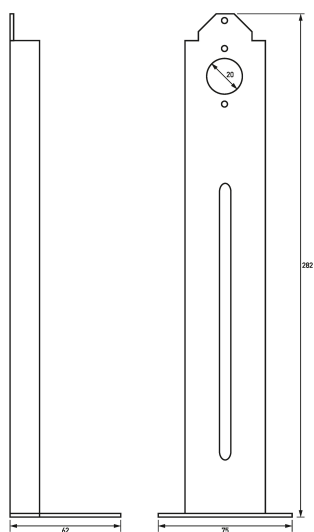
Maßzeichnung Montagesätze SIWH
