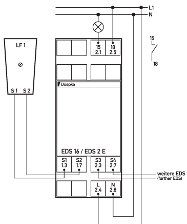
Anschlusschema
