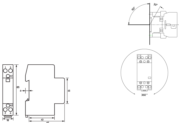
Maßzeichnung Installationsschütze HS 1-024AC/25-20
