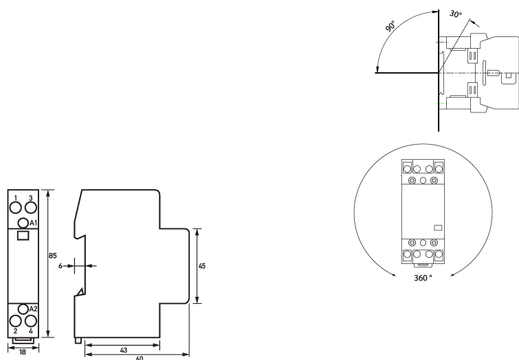
Maßzeichnung Installationsschütze HS 1-230AC/20-10
