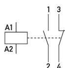
Schaltungsbeispiel Installationsschütze HS 1-230AC/20-11
