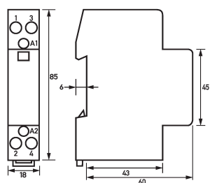
Maßzeichnung Installationsschütze HS 1-230AC/20-20
