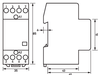
Maßzeichnung Installationsschütze HS 2-024AC/25-40
