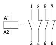
Schaltungsbeispiel Installationsschütze HS 2-230AC/24-13
