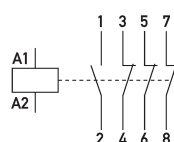
Schaltungsbeispiel Installationsschütze HS 2-230AC/24-13
