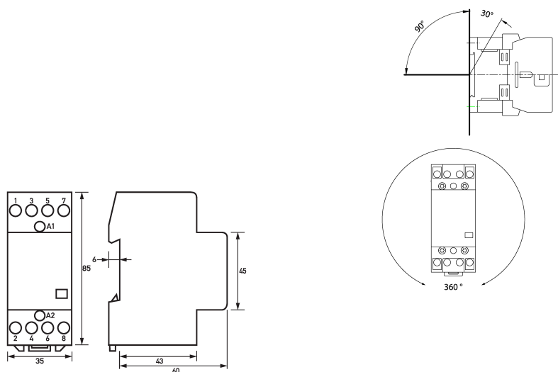
Maßzeichnung Installationsschütze HS 2-230AC/24-13
