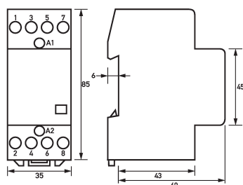
Maßzeichnung Installationsschütze HS 2-230AC/25-04
