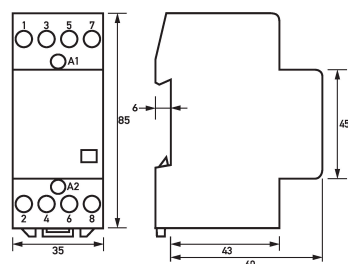
Maßzeichnung Installationsschütze HS 2-230AC/25-13
