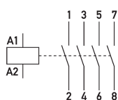
Schaltungsbeispiel Installationsschütze HS 2-230AC/25-40
