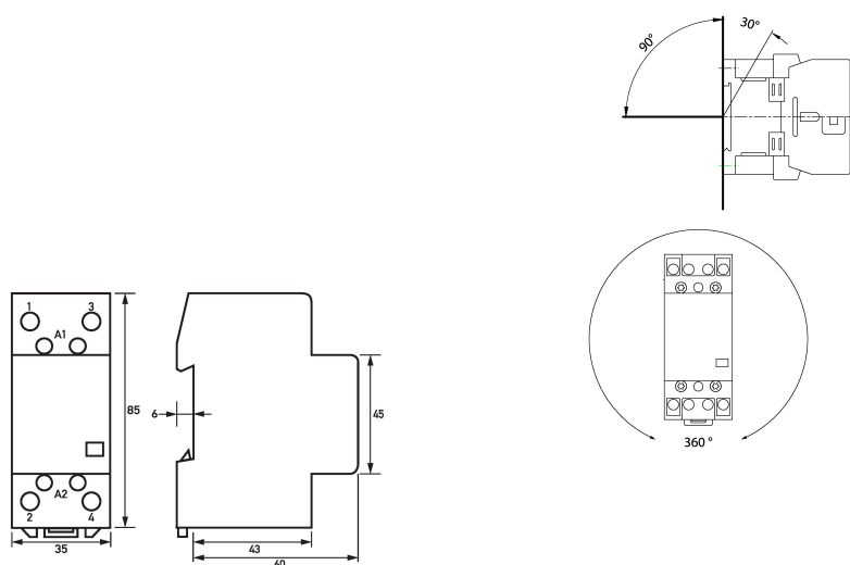
Maßzeichnung Installationsschütze HS 2-230AC/40-20S
