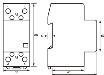
Maßzeichnung Installationsschütze HS 2-230AC/63-20S
