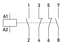
Schaltungsbeispiel Installationsschütze HS 2-230UC/25-22
