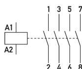
Schaltungsbeispiel Installationsschütze HS 2-230UC/25-40
