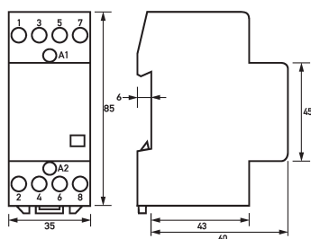
Maßzeichnung Installationsschütze HS 2-230UC/25-40
