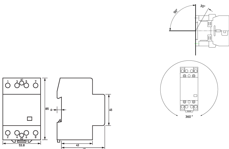
Maßzeichnung Installationsschütze HS 3-024AC/63-22
