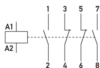
Schaltungsbeispiel Installationsschütze HS 3-024AC/63-22
