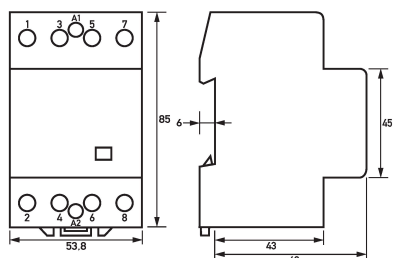
Maßzeichnung Installationsschütze HS 3-024AC/63-40
