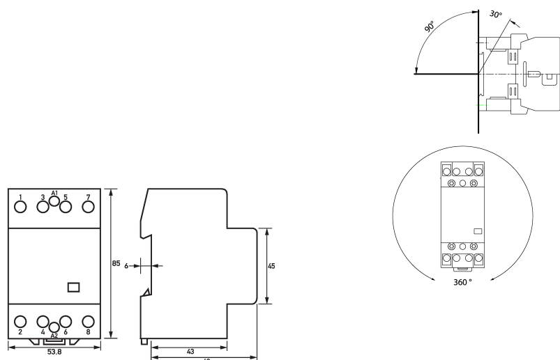
Maßzeichnung Installationsschütze HS 3-230AC/40-22
