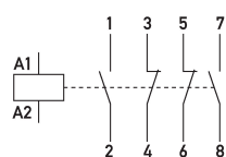
Schaltungsbeispiel Installationsschütze HS 3-230AC/40-22
