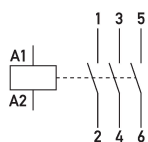
Schaltungsbeispiel Installationsschütze HS 3-230AC/40-30
