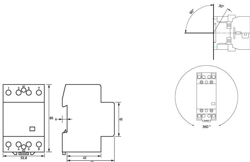
Maßzeichnung Installationsschütze HS 3-230AC/40-30
