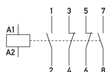
Schaltungsbeispiel Installationsschütze HS 3-230AC/63-22
