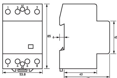
Maßzeichnung Gruppenansicht
