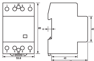
Maßzeichnung Installationsschütze HS 3-230AC/63-22
