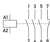
Schaltungsbeispiel Installationsschütze HS 3-230AC/63-31
