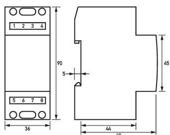
Maßzeichnung Gruppenansicht
