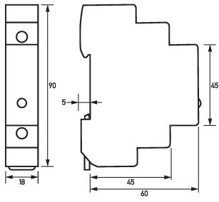
Maßzeichnung Gruppenansicht
