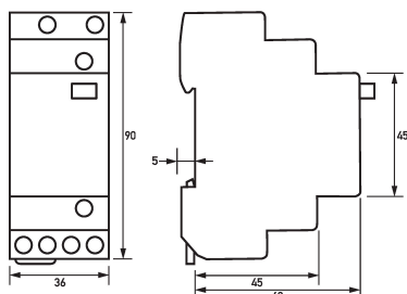
Maßzeichnung Gruppenansicht
