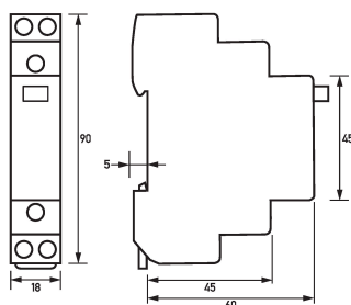
Maßzeichnung Stromstoßschalter (Fernschalter) RS 012-100
