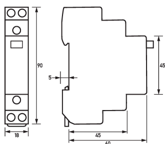
Maßzeichnung Stromstoßschalter (Fernschalter) RS 012-100
