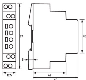
Maßzeichnung Treppenlichtzeitschalter RTZ 2
