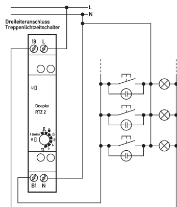
Schaltungsbeispiel Treppenlichtzeitschalter RTZ 2
