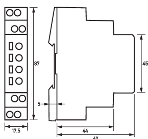
Maßzeichnung Gruppenansicht
