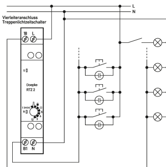
Anschlusschema
