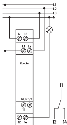
Schaltungsbeispiel Unterspannungsmessrelais RUR 3
