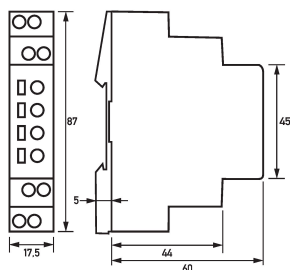
Maßzeichnung Unterspannungsmessrelais RUR 3
