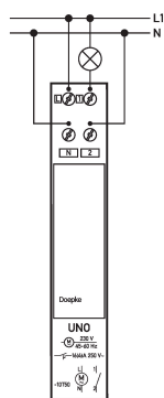
Schaltungsbeispiel Zeitschaltuhren Uno QRD
