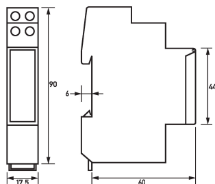
Maßzeichnung Zeitschaltuhren Uno QRD
