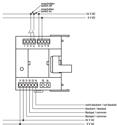
Schaltungsbeispiel automatisch wiedereinschaltende Einrichtungen DFA 2-2
