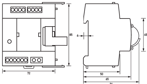
Maßzeichnung automatisch wiedereinschaltende Einrichtungen DFA 2-2
