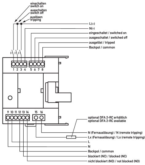
Schaltungsbeispiel automatisch wiedereinschaltende Einrichtungen DFA 2-3
