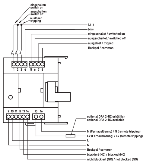
Anschlusschema
