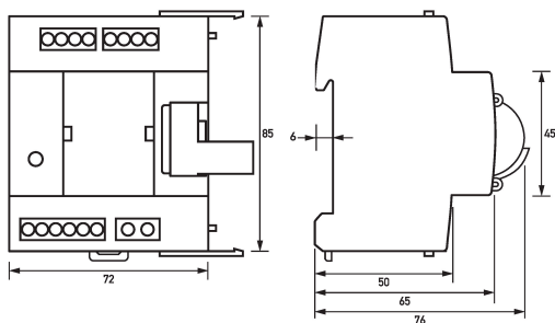
Maßzeichnung automatisch wiedereinschaltende Einrichtungen DFA 2-3
