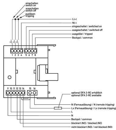
Anschlusschema
