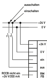
Schaltungsbeispiel automatisch wiedereinschaltende Einrichtungen DFA 3 024DC-0
