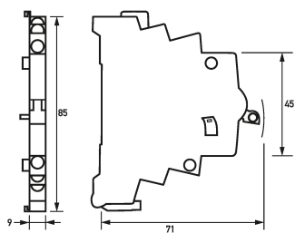
Maßzeichnung Störmeldefhlfsschalter DHi-S10
