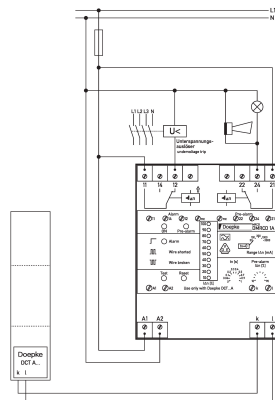
Anschlussschema
