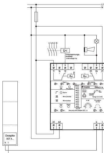
Anschlusschema
