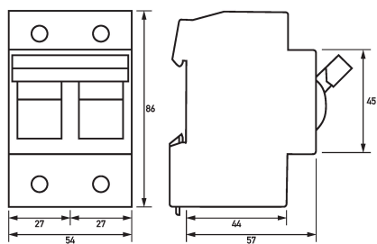
Maßzeichnung Gruppenansicht
