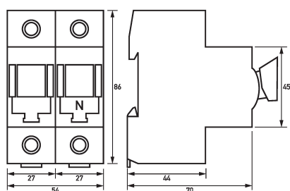
Maßzeichnung Gruppenansicht
