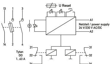
Anschlusschema
