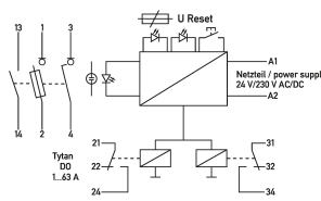
Anschlussschema
