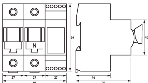
Maßzeichnung Gruppenansicht
