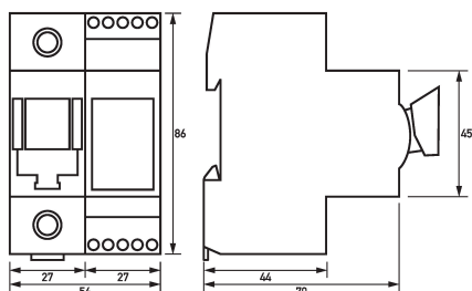
Maßzeichnung Gruppenansicht
