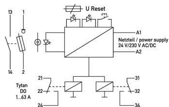
Anschlusschema
