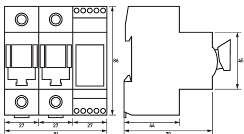
Maßzeichnung Gruppenansicht
