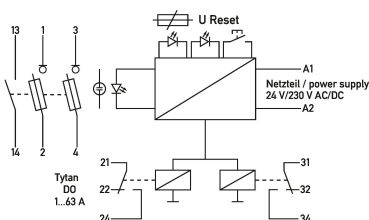
Anschlusschema
