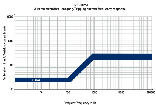
Diagramme Fehlerstromschutzschalter DFS 2 016-2/0,03-B NK
