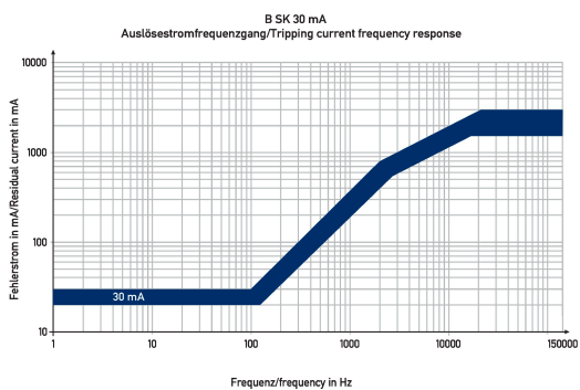
Diagramme Fehlerstromschutzschalter DFS 2 016-2/0,03-B SK
