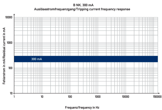
Diagramme Fehlerstromschutzschalter DFS 2 016-2/0,30-B NK
