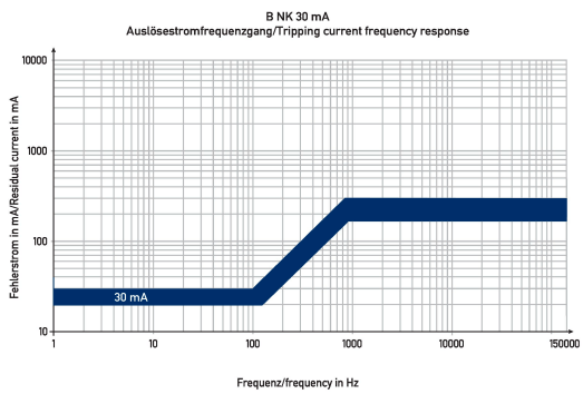
Diagramme Fehlerstromschutzschalter DFS 2 040-2/0,03-B NK
