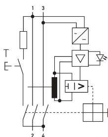
Schaltungsbeispiel Fehlerstromschutzschalter DFS 2 040-2/0,30-B NK
