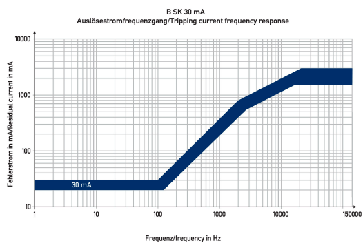
Diagramme Fehlerstromschutzschalter DFS 2 063-2/0,03-B SK
