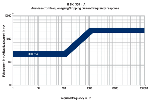
Diagramme Fehlerstromschutzschalter DFS 2 063-2/0,30-B SK
