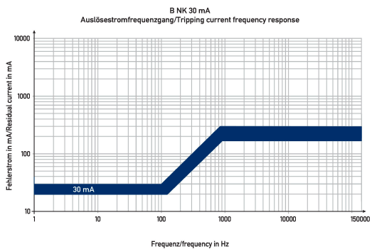
Diagramme Fehlerstromschutzschalter DFS 2 080-2/0,03-B NK
