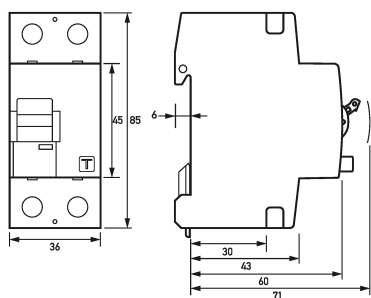
Maßzeichnung Fehlerstromschutzschalter DFS 2 125-2/0,10-A KV
